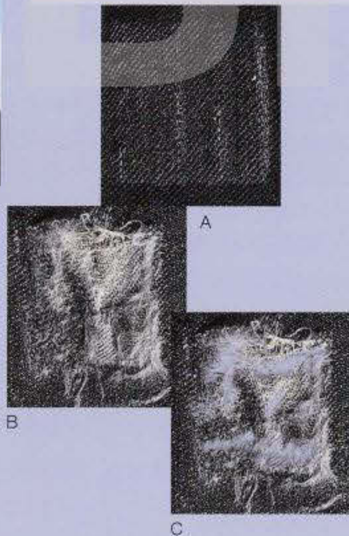
Abriebergebnisse im Vergleich: A. InoTex B. Kepritec Jeans C. Jeans
